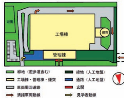
工場配置図
